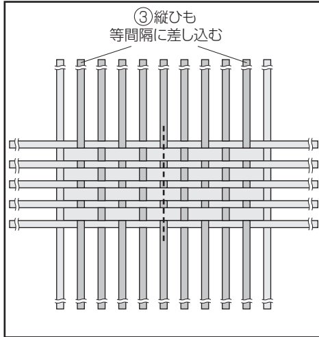
5 残りの縦ひも③を図のように等間隔になるように交互に差し込みます。この時の縦ひも③は差し込むだけでボンドでは止めません。
